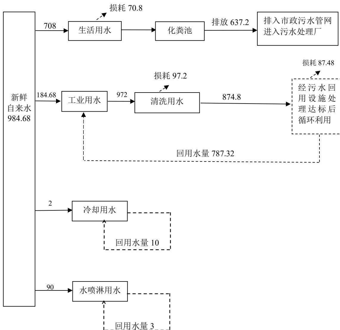
图3 项目水平衡图 单位：m 3 /a
