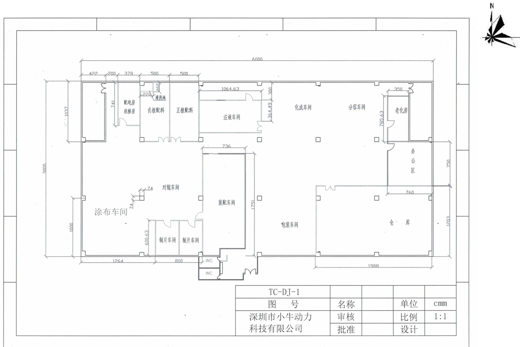
附图 11-2 项目 A1 栋厂房平面布置图
