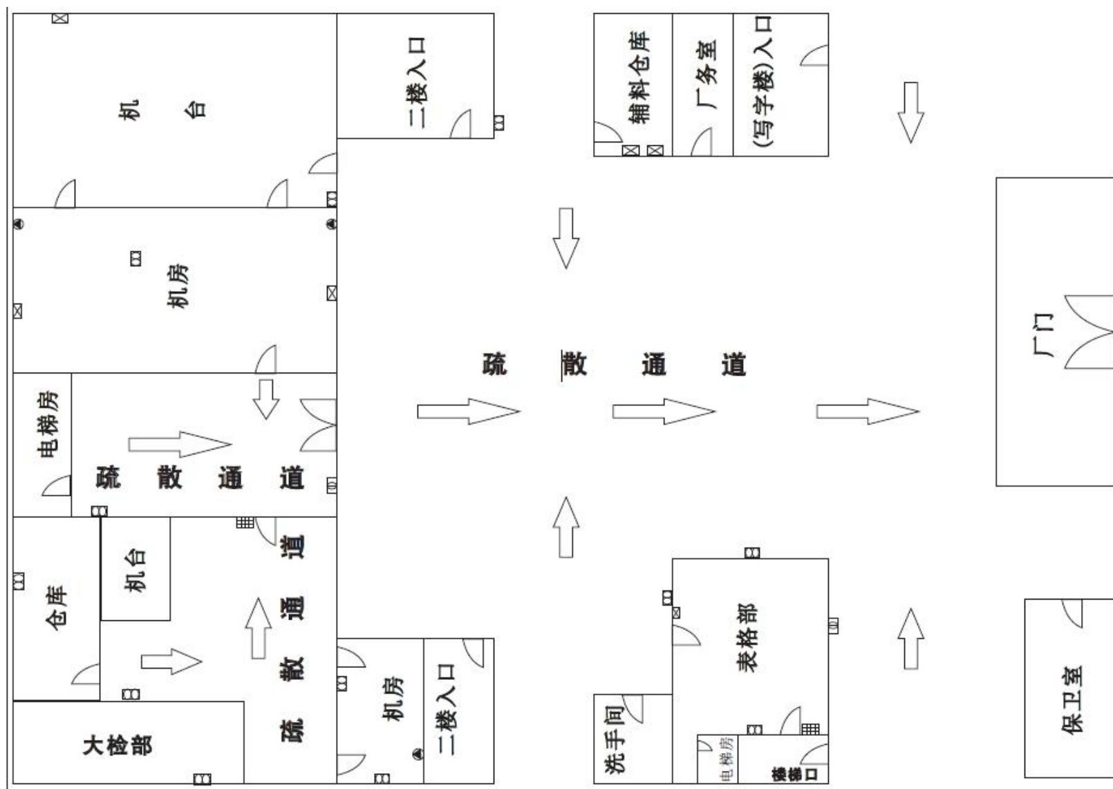
附图 5-1 项目车间平面布置图 (1F)
