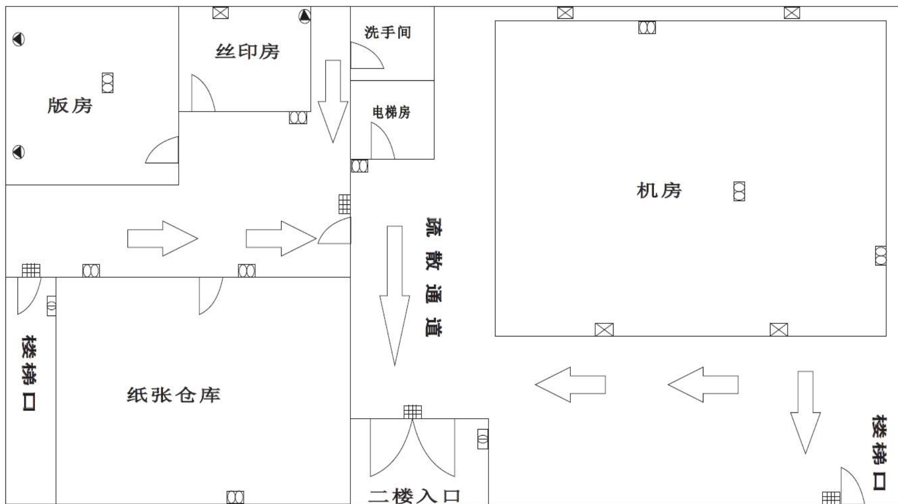
附图 5-2 项目车间平面布置图（2F）
